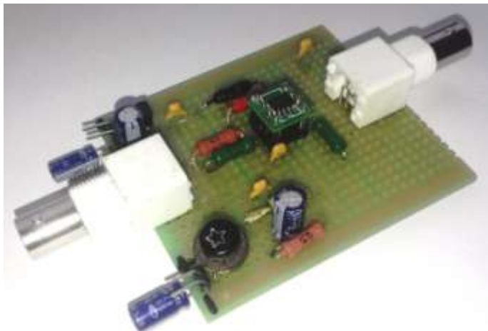
Широкопasmовий підсилювач UWB сигналу на базі операційного підсилювача AD8045
