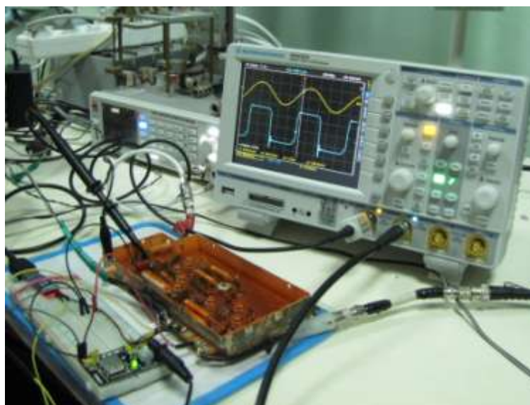
Формувач імпульсів запуску на тунельному діоді 3И306Н для генератора UWB
