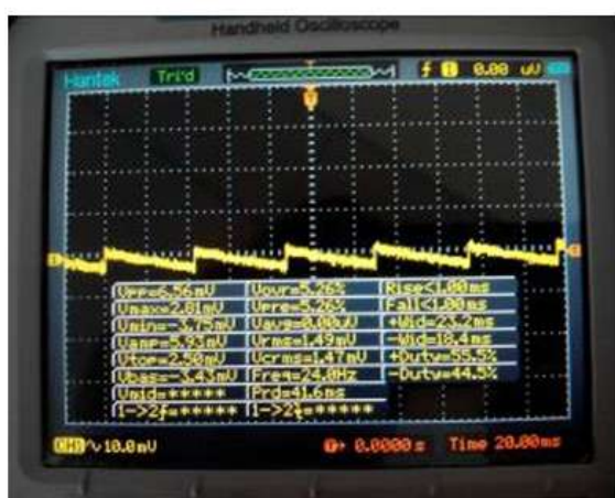
Перевірка входних та вихідних перетворювачів та системи в цілому (канал-шина 5 V)
